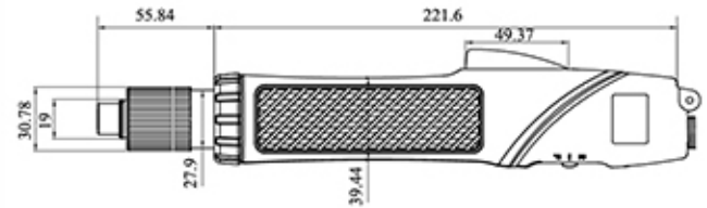
SKD-BN800L
